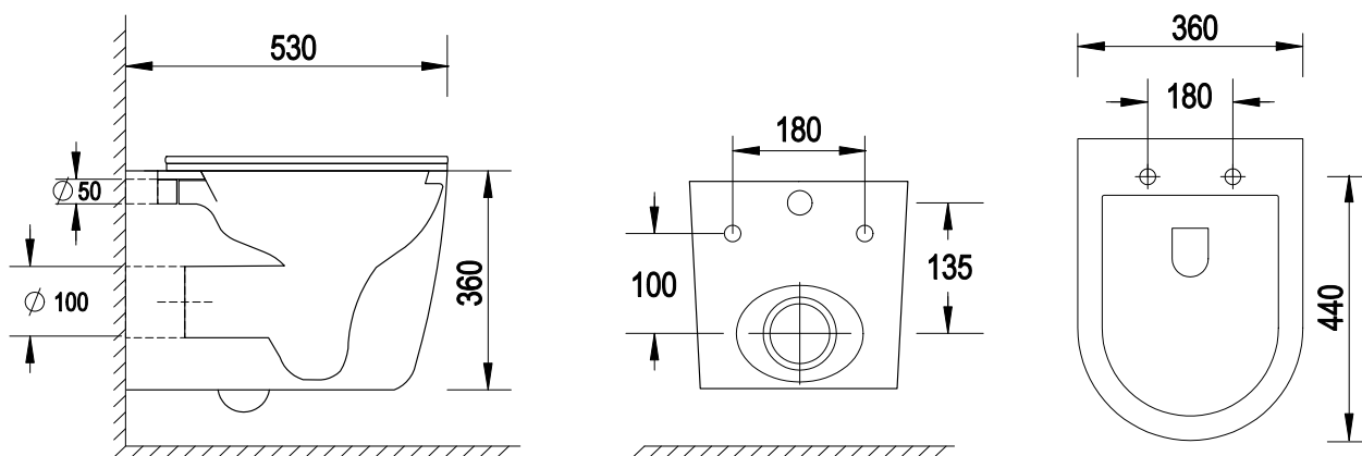
RYСУNEK TECHNICZNY
