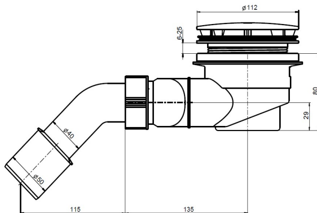
Rysunek techniczny
